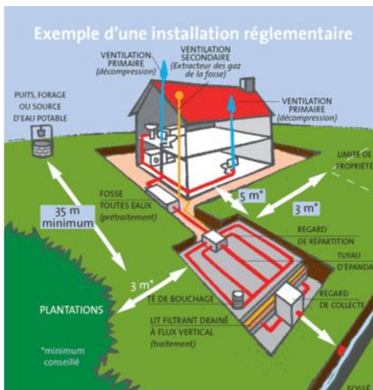
Schéma récapitulatif d'une installation d'assainissement non collectif réglementaire
